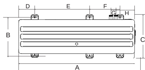
8/10/12/16 kW (unità:mm)
