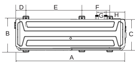
4/6 kW (unità:mm)
